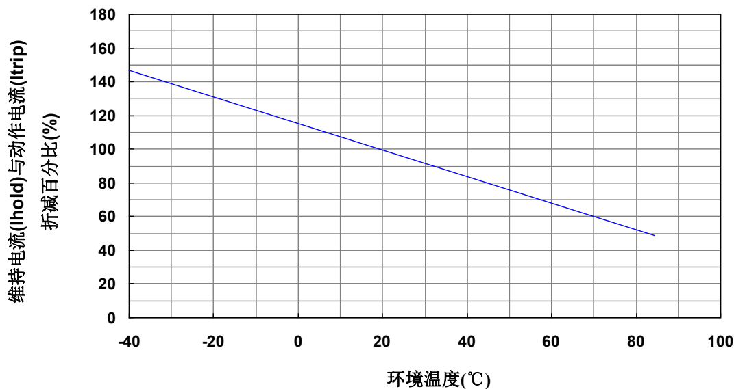
KMC3S (1206)系列
